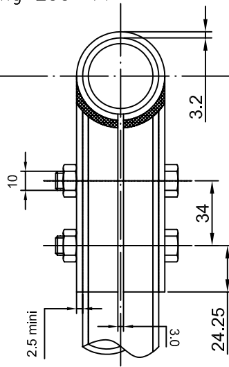
Dessin/Drawing 253-46
